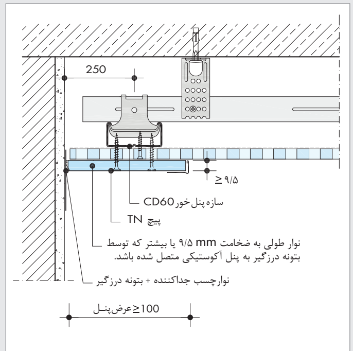
اتصال به دیوار بنایی با حاشیه پله‌ای
